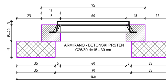
PRESJEK 1-1 M 1:20
