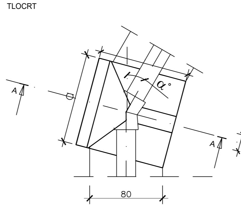
HORIZONTALNI LOM NIVELETE CJEVOVODA
