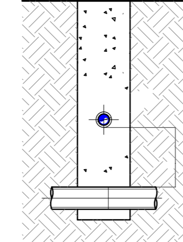
Križanje kanalizacije i vodovod - tipski detalj
