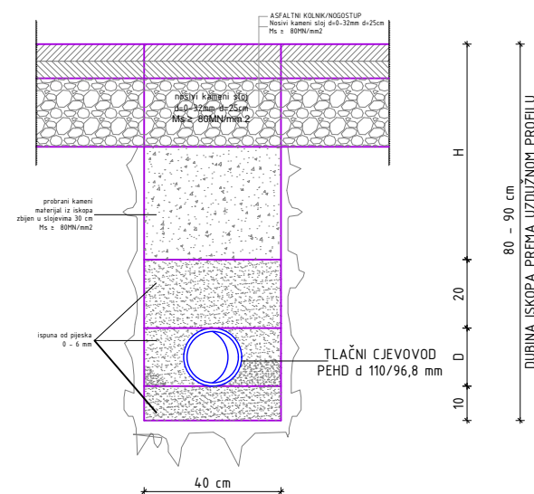
NORMALNI PRESJEK ROVA ZA CJEVOVOD PEHD d110 mm
