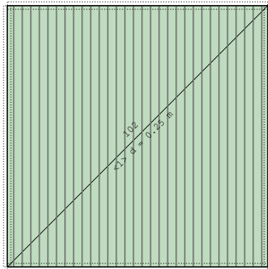
Nivo: temeljna ploča [0.00 m]
