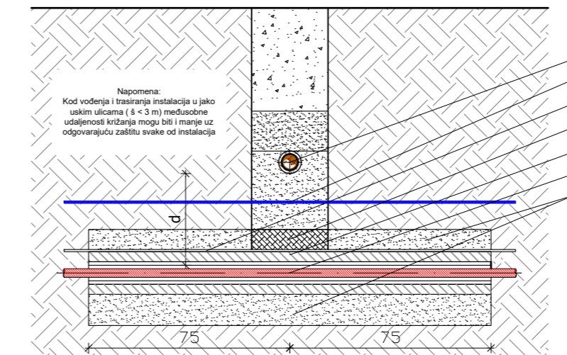
Križanje EKI instalacije i vodovoda
