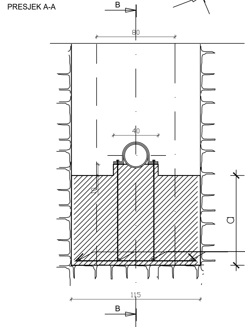
OGRLICA OD PLOŠNOG ŽELJEZA 80/10mm, L=95 cm kom.1 MJ 1:5
