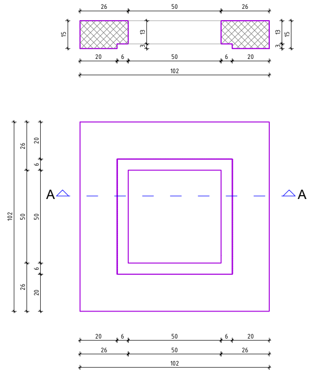
DETALJ AB PLOČE SLIVNIČKE REŠETKE M 1:20
